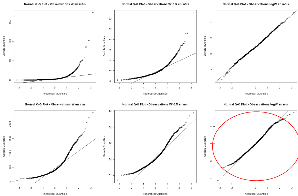
Figure 5 : QA observé - QQplot après différentes transformations
