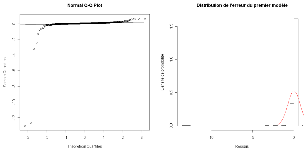
Figure 17 : Distribution de l'erreur du premier modèle – QA
