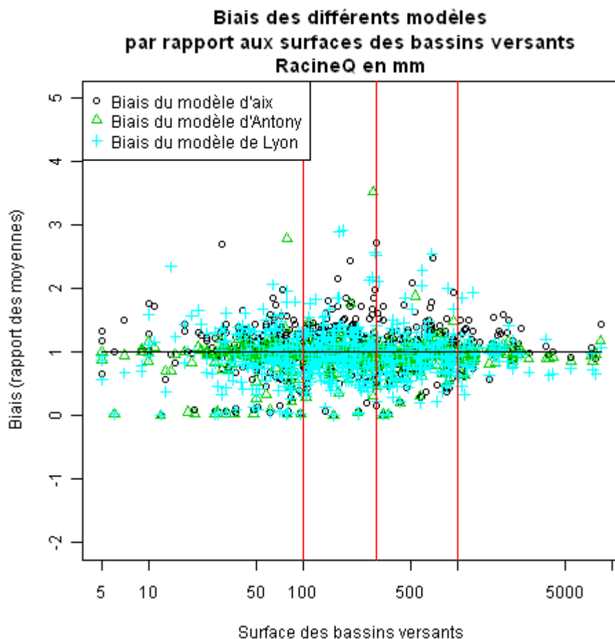
Figure 9 : Biais des différents modèles de QMNA5 (RacineQ en mm/mois)
