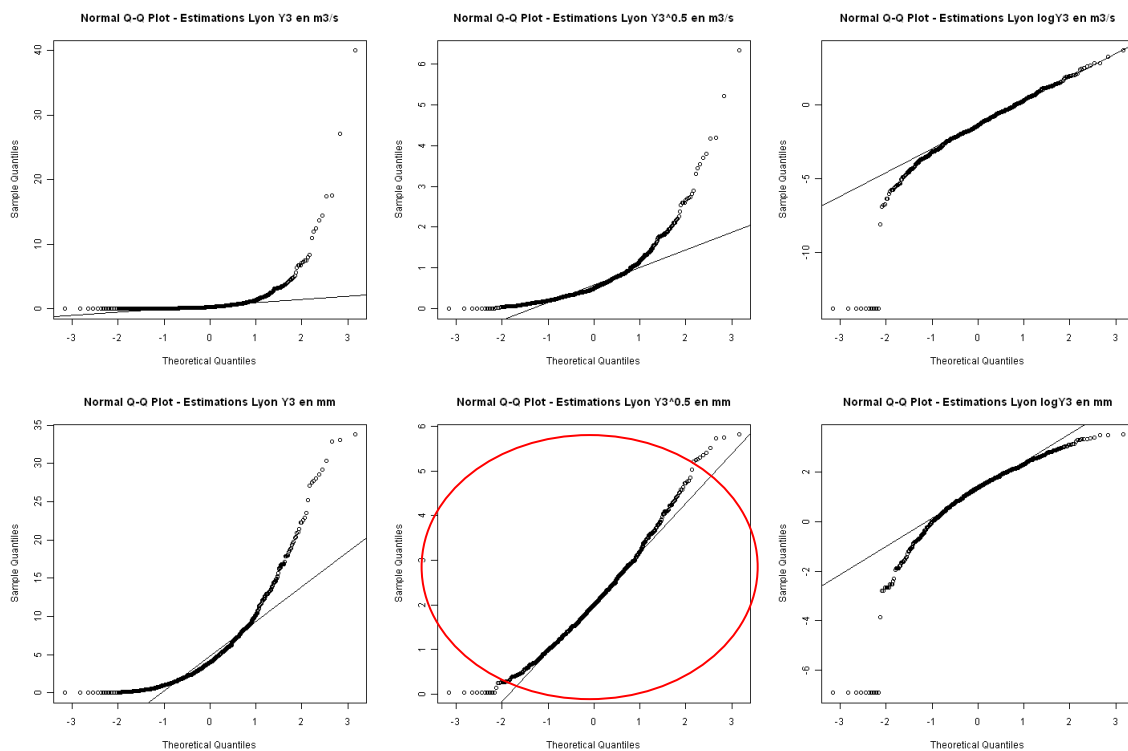
Figure 4 : QMNA5 Estimations du modèle CART- QQplot après différentes transformations
