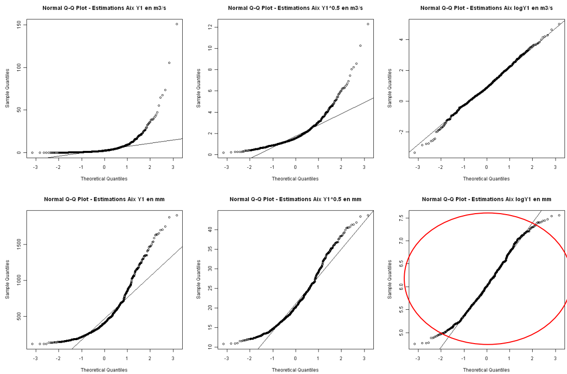
Figure 6 : QA Estimations du modèle pluie-débit - QQplot après différentes transformations de la variable
