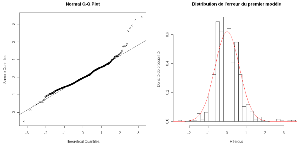
Figure 16 : Distribution de l'erreur du premier modèle - QMNA5
