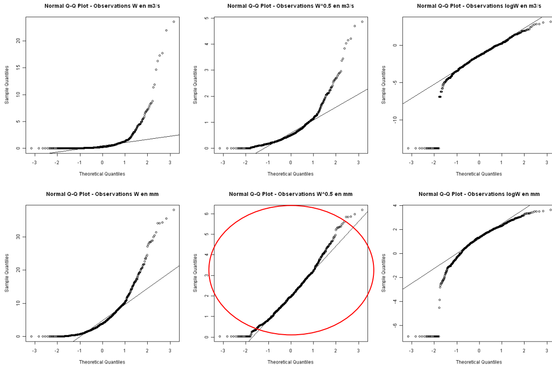
Figure 1 : QMNA5 observé - QQplot après différentes transformations
