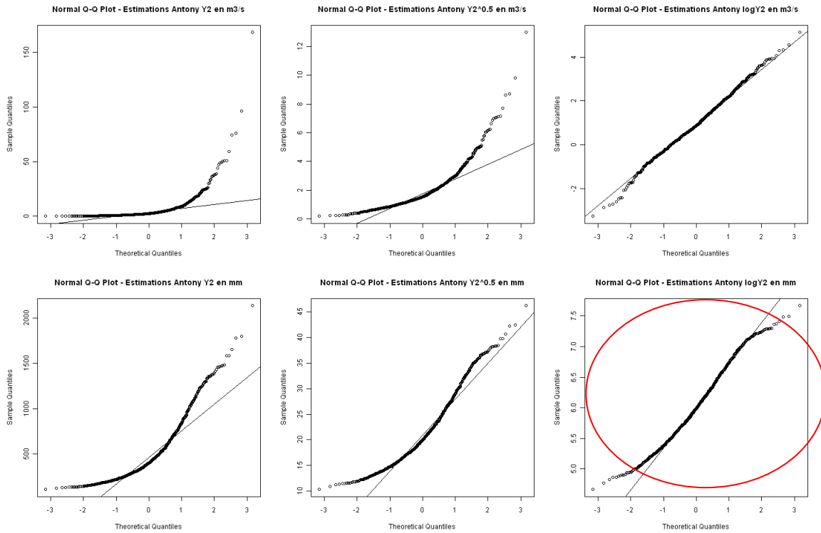
Figure 7 : QA Estimations du modèle IDW - QQplot après différentes transformations
