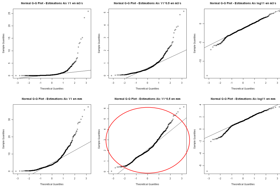
Figure 2 : QMNA5 Estimations issues du modèle pluie-débit - QQplot après différentes transformations
