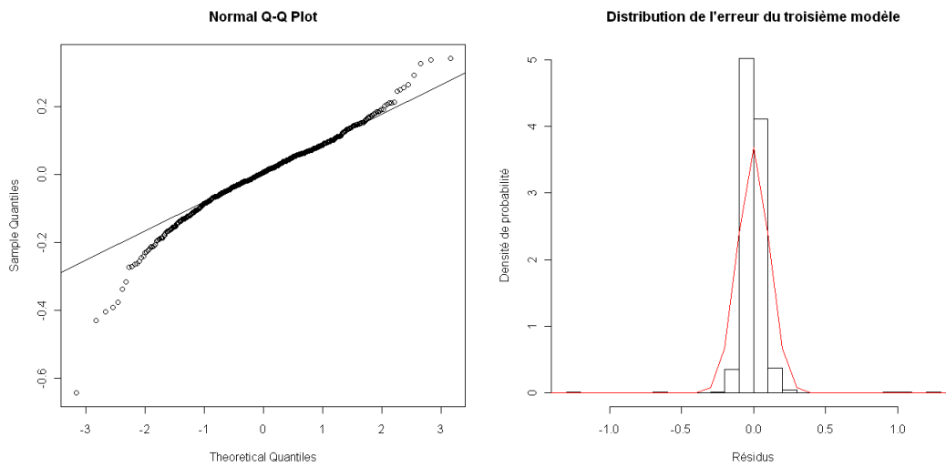
Figure 23 : Distribution de l'erreur du troisième modèle - Q_a
