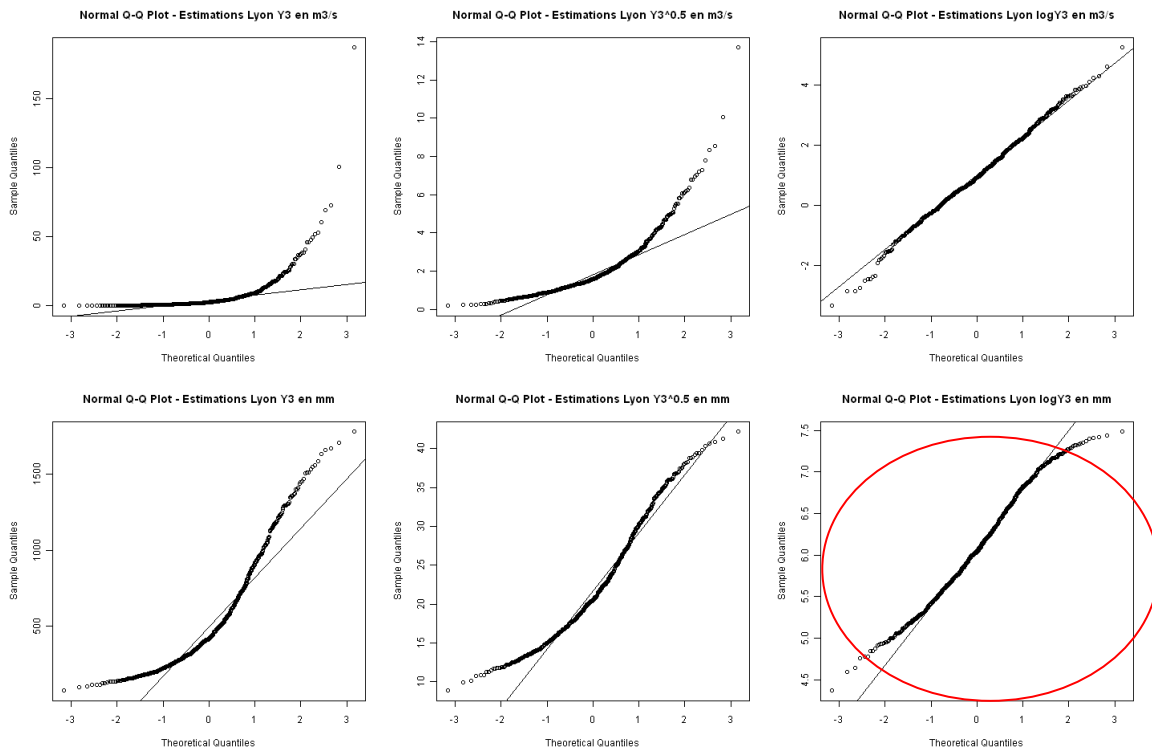
Figure 8 : QA Estimation du modèle CART - QQplot après différentes transformations
