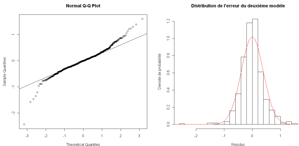
Figure 19 : Distribution de l'erreur du deuxième modèle - QMNA5
